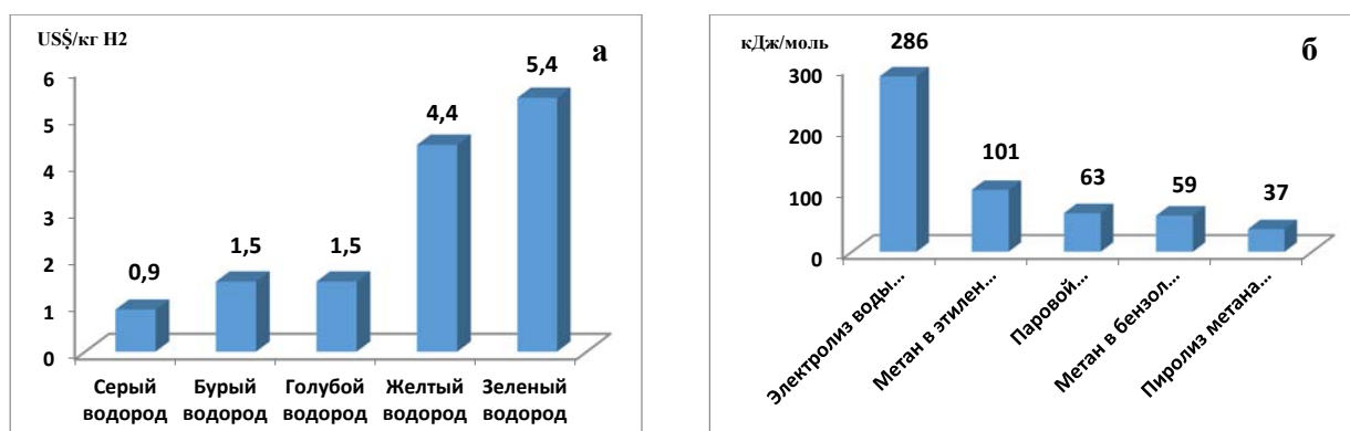
Рис. 2. Стоимость производства различных видов водорода (а) и затраты энергии на образование водорода в различных процессах (б).
