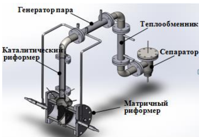
Рис. 7. 3D-схема демонстрационной установки комбинированного матричного и каталитического риформинга для получения водорода.
