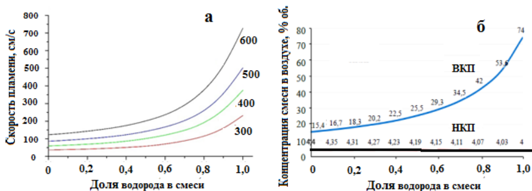
Рис. 6. Зависимость от объемной доли водорода в метановодородной смеси (а) ламинарной скорости пламени при разной начальной температуре (К), (б) нижнего концентрационного предела (НКП) и верхнего концентрационного предела (ВКП) распространения пламени (по материалам [14] и [18]).
