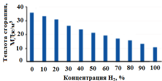
Рис. 4. Зависимости теплоты сгорания метановодородных смесей от концентрации водорода.
