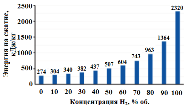
Рис. 5. Зависимость затрат энергии на сжатие метановодородной смеси давлением 1 МПа от концентрации в ней водорода (по материалам [14]).
