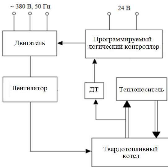
Рис. 2. Функциональная схема автоматической системы управления твердотопливного котла.
