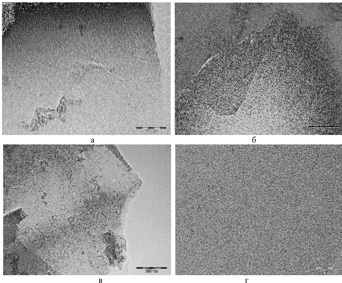
Рисунок 5 – ПЭМ снимки графена
