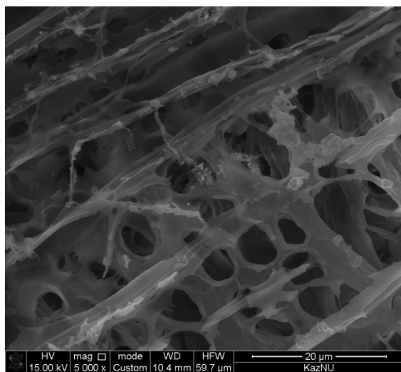
Рис. 2 – SEM-изображения образца
