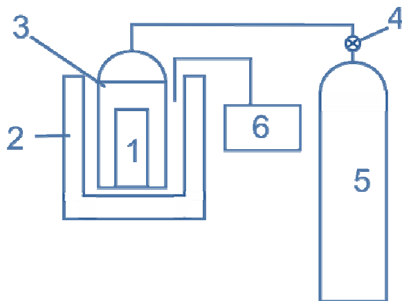
1 – алундовый тигель, 2 – муфельная печь, 3 – стальной стакан, 4 – игольчатый кран, 5 – баллон с аргонем, 6 – контроллер температуры
