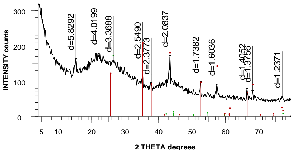
Рис. 3 – Рентгенограмма полученного образца КРШ
