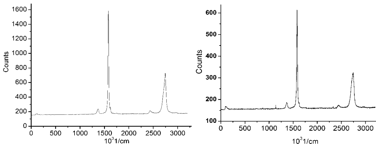
Рис. 4 – Рамановские спектры графена
